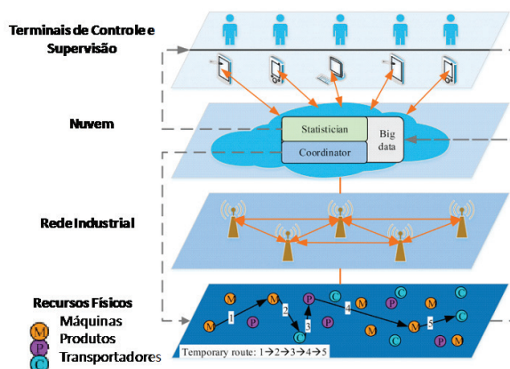
Figura 3. Representação esquemática de uma fábrica inteligente da indústria 4.0.
