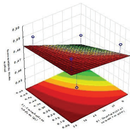
Figura 4. (a) Superfície resposta para o modelo linear da variável nitrato residual. X2- concentração de nitrato em g/L, X1- Concentração de corante em ppm.
